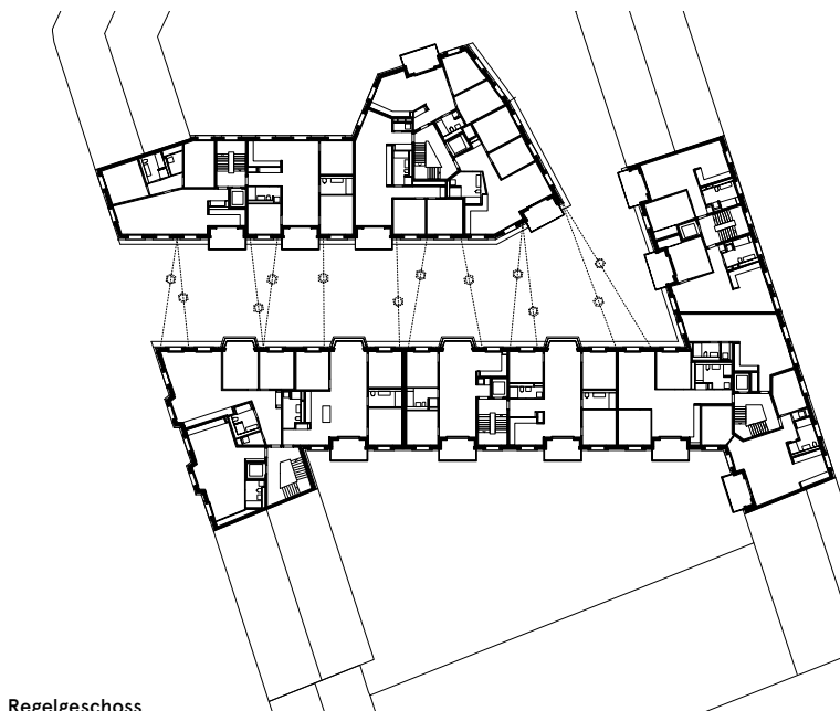
Regelgeschoss
